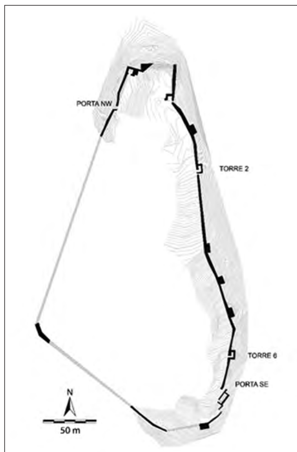
FIGURA 32. Planta del jaciment del Puig del Castell de Samalús. Font: Elaboració pròpia.
